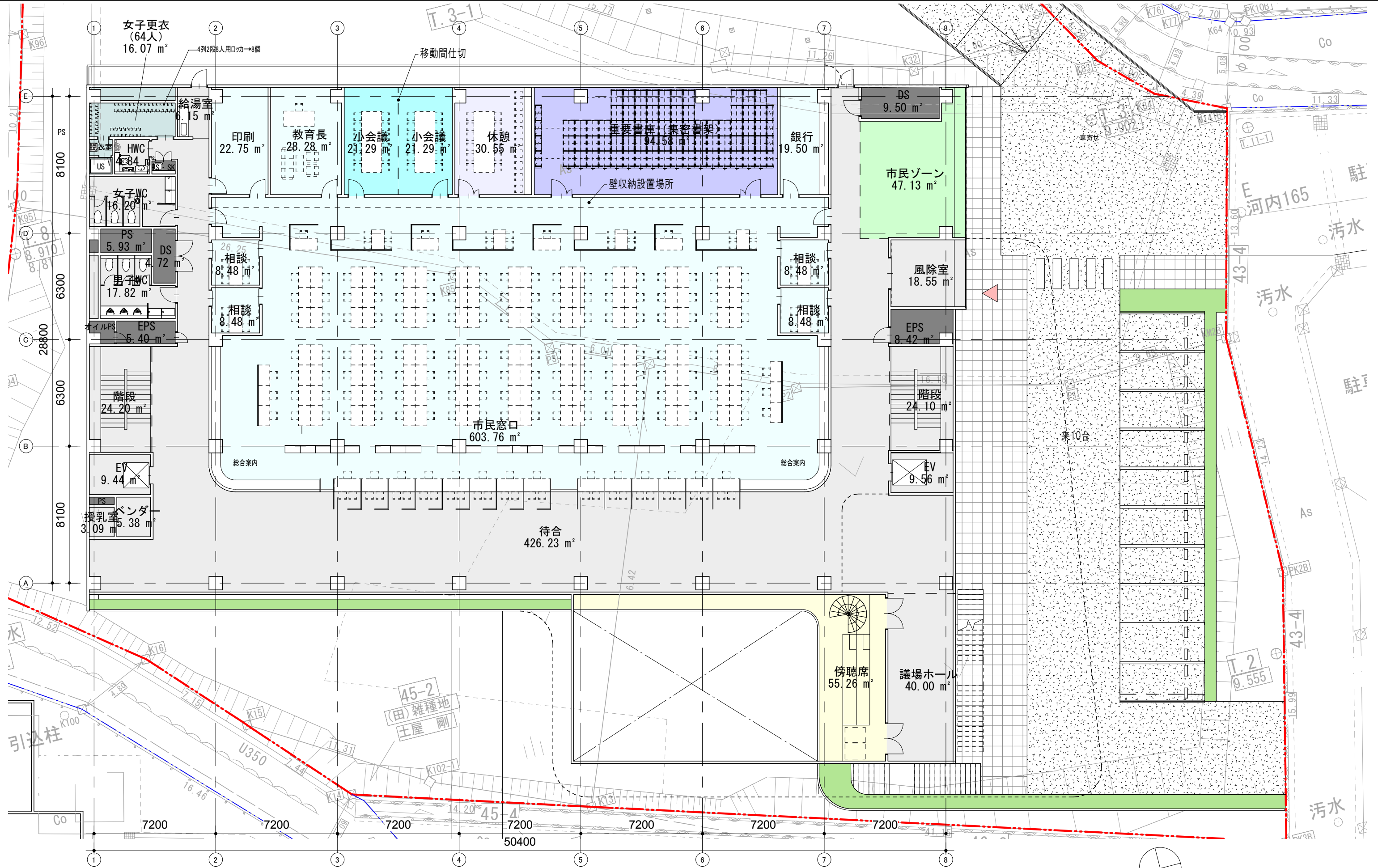
2F平面図 200
